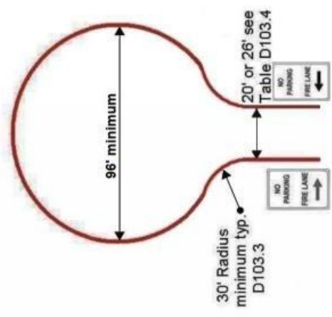
Cul-De-Sac
